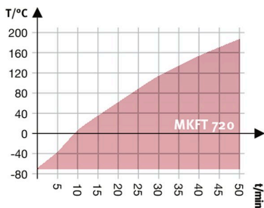
Кривая нагрева
